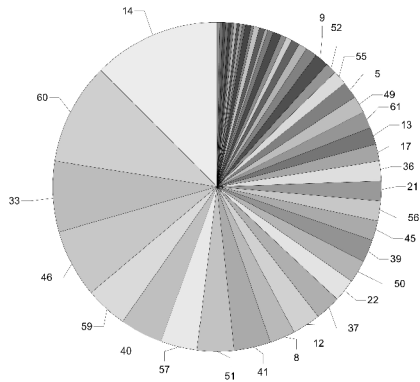
Incidenza dei tipi paesaggistici
